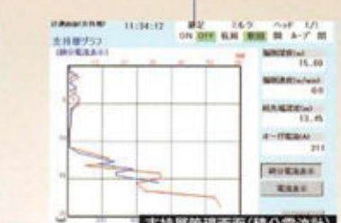
■支持層管理画面(積分電流計) 積分電流値により、地盤状況を把握できます。
